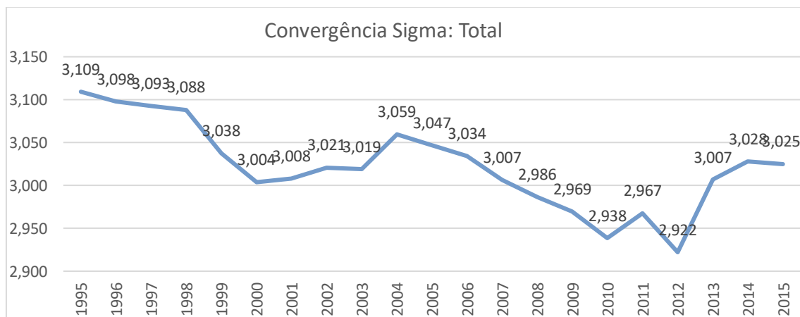
Gráfico 6- Convergência Sigma aplicada ao total das indústrias (EU28)
