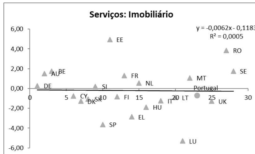
Gráfico A.3.3.2 – Convêrgencia Beta aplicada ao setor Imobiliário
